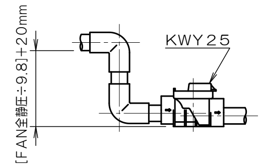
封水高さの取り方
